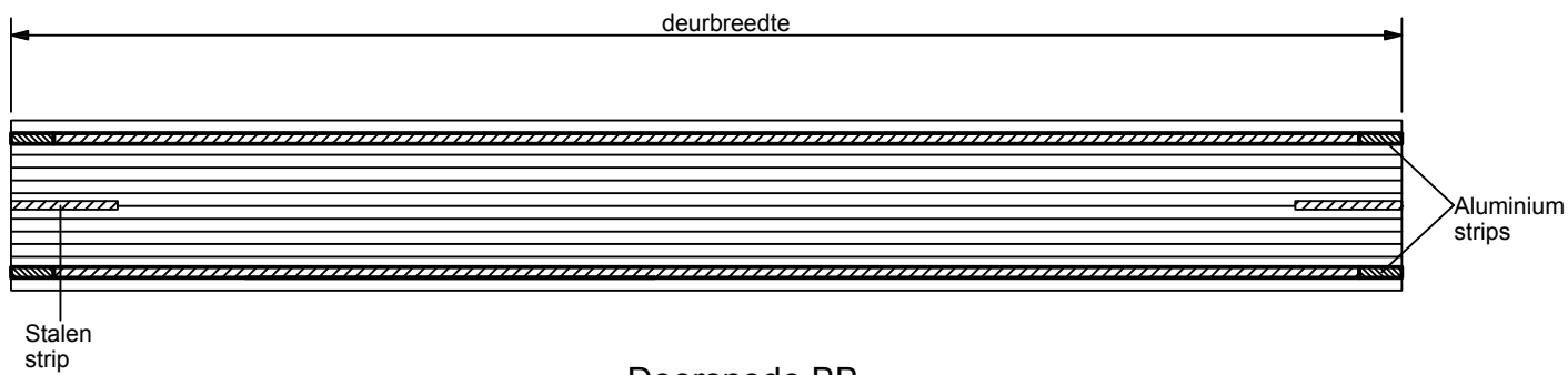
Doorsnede BB
