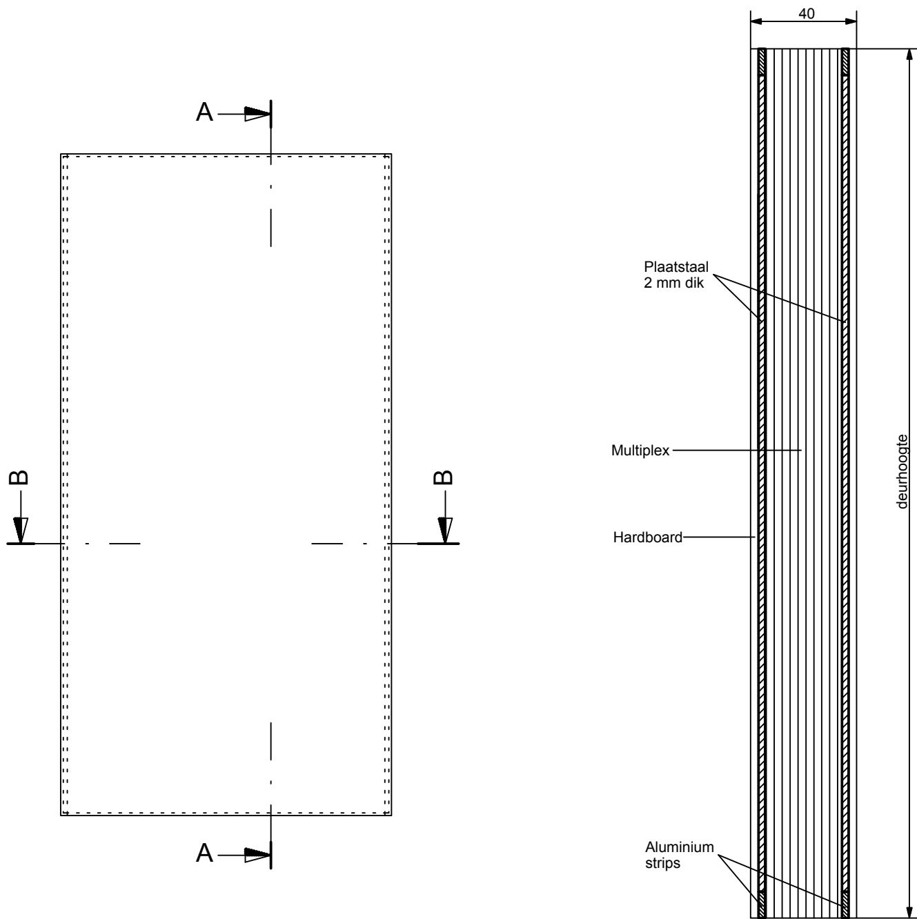
Doorsnede AA
