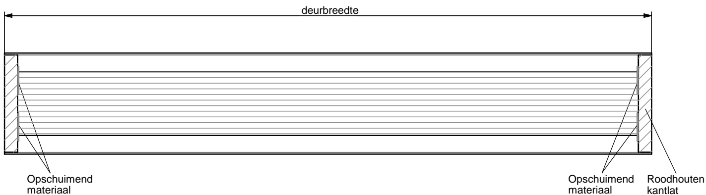
Doorsnede BB
