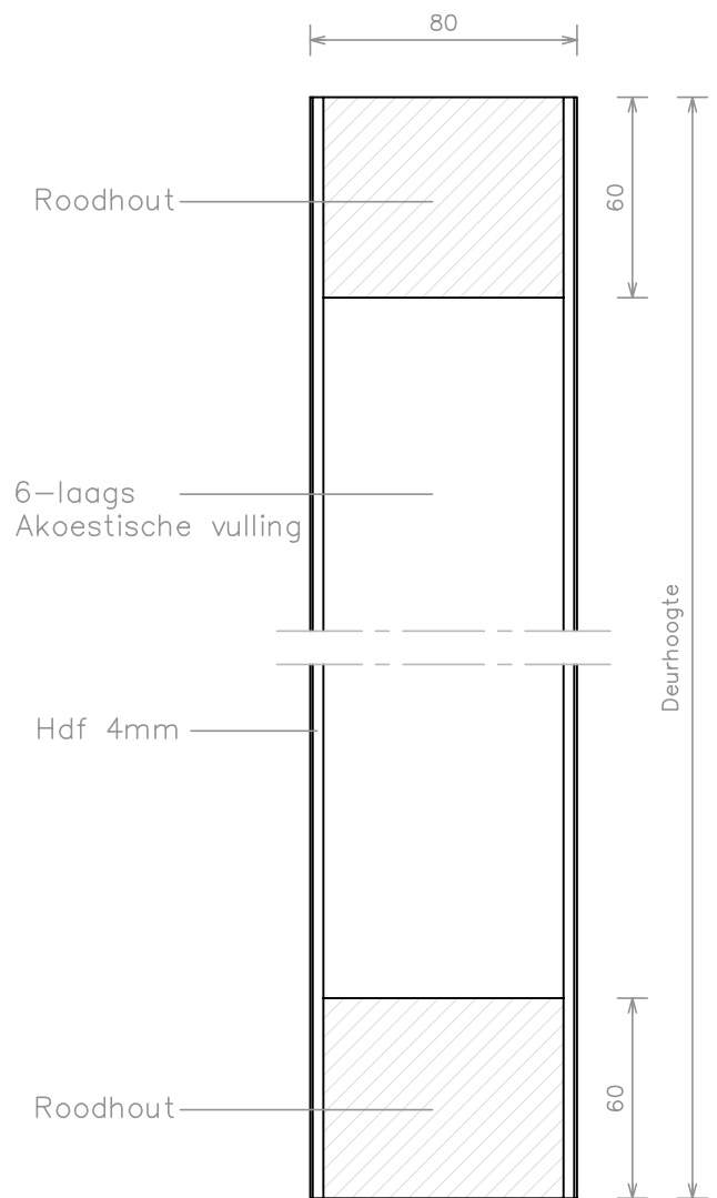
Doorsnede AA
