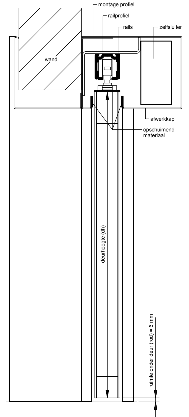
DOORSNEDE AA
