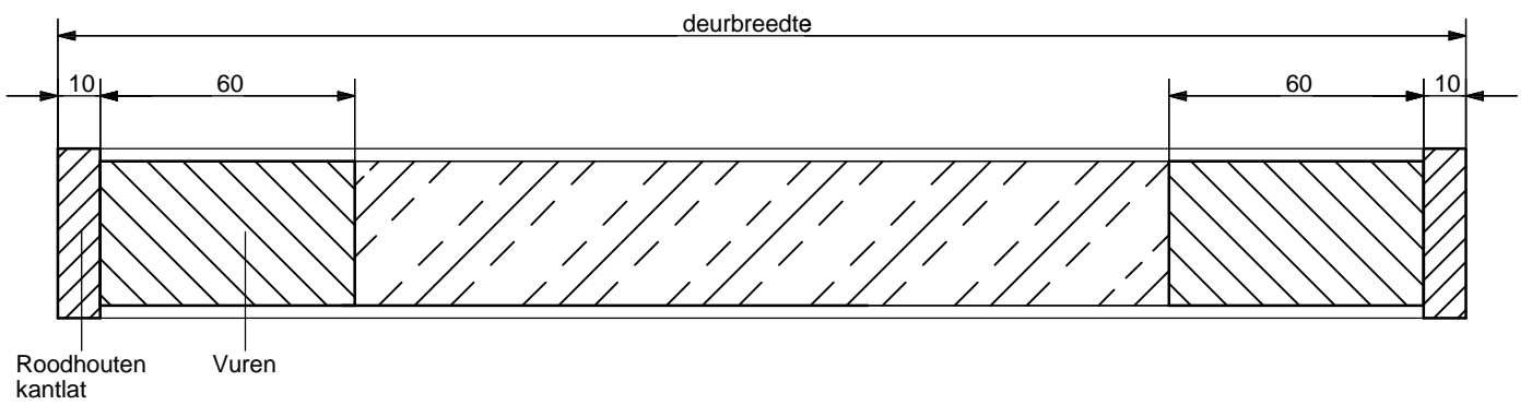
Doorsnede BB
