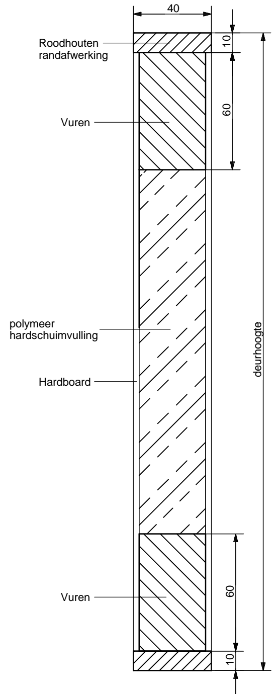
Doorsnede AA
